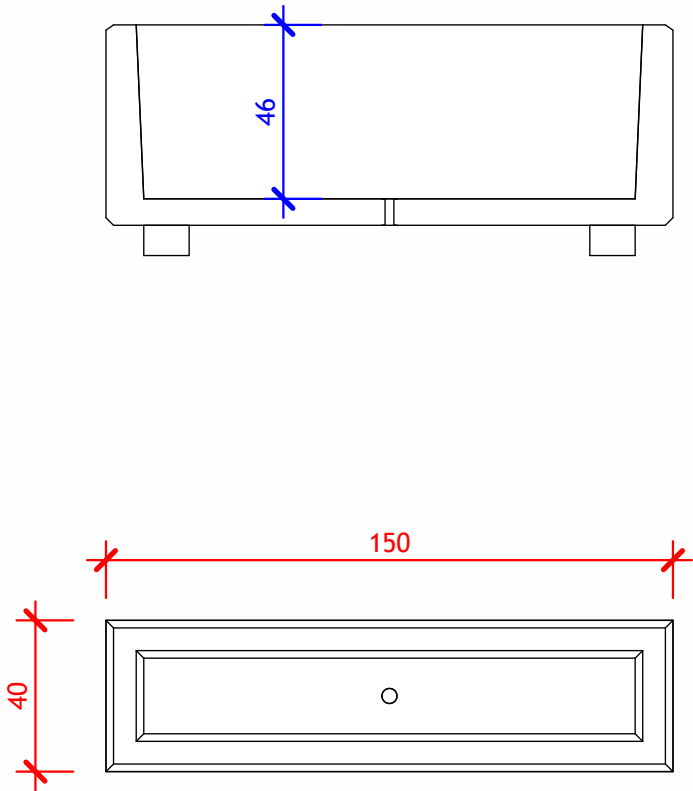
BAC A FLEUR BETON 2 PIEDS 134L - Vue en plan
