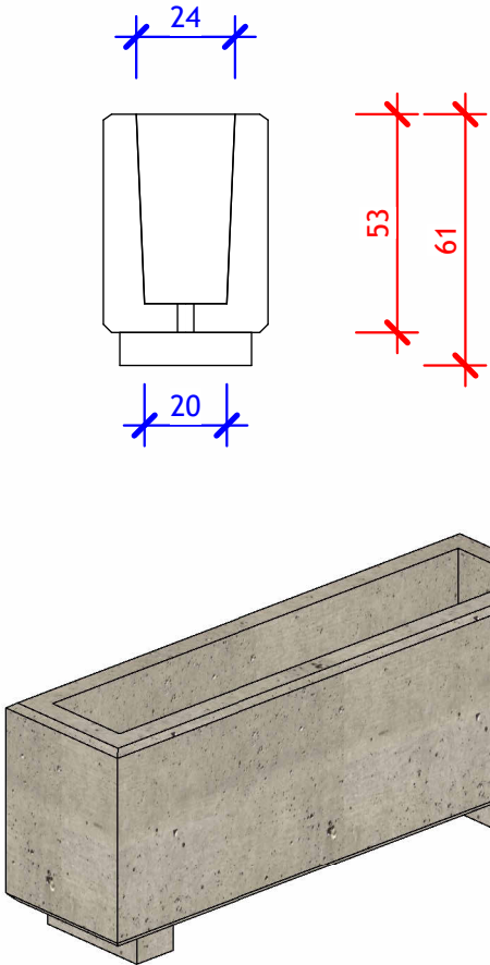
BAC A FLEUR BETON 2 PIEDS 134L - Vue 3D
