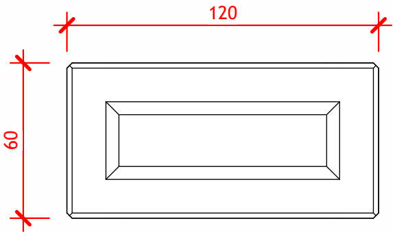
BAC A FLEUR BETON 128L - Vue en plan
