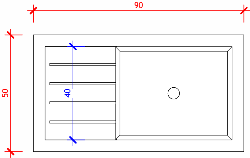
EVIER BETON 64L EGOUTTOIR- Vue en plan
