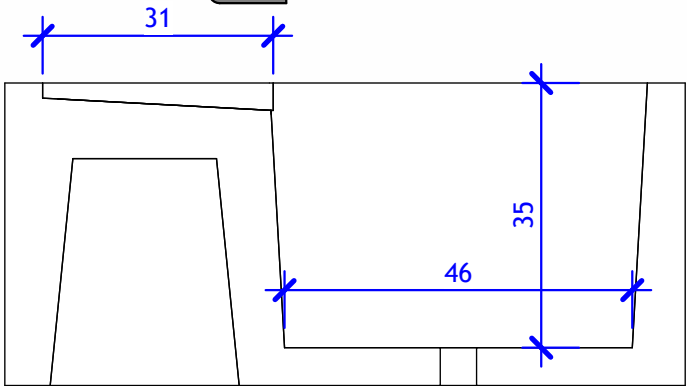
EVIER BETON 64L EGOUTTOIR - Coupe longitudinale
