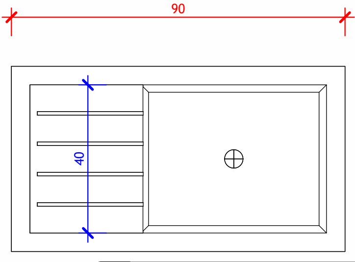
EVIER BETON EGOUTTOIR 27L - Vue en plan
