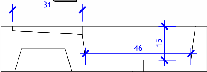
EVIER BETON EGOUTTOIR 27L - Coupe longitudinale
