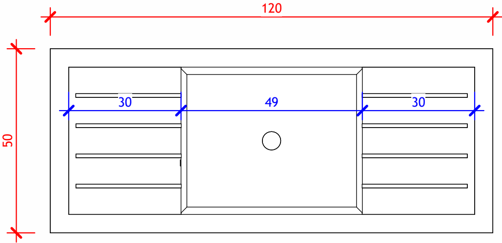
EVIER BETON DOUBLE EGOUTTOIR 27L- Vue en plan
